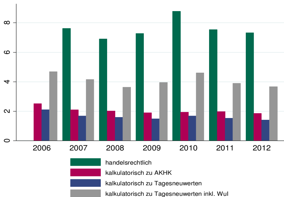
Abbildung 4-20 Investitionsquote der Gas-Verteilnetzbetreiber (arithmetische Mittelwerte in Prozent)
