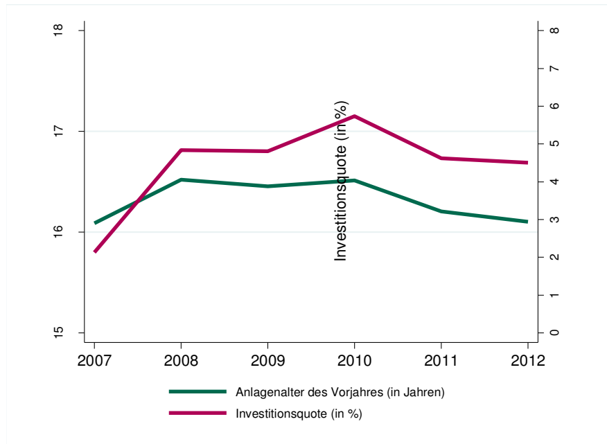
Abbildung 4-34 Zeitliche Entwicklung von Anlagenalter und Investitionsquote der (arithmetische Mittelwerte basierend auf 3 Übertragungsnetzbetreibern)
