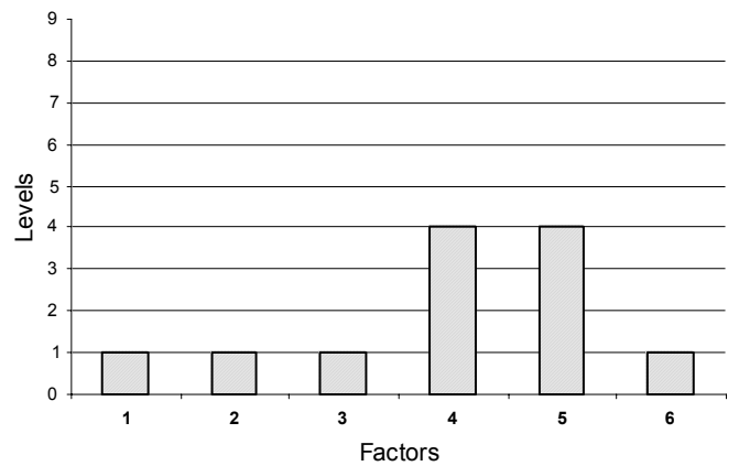
AIFAI \leq 5.17
