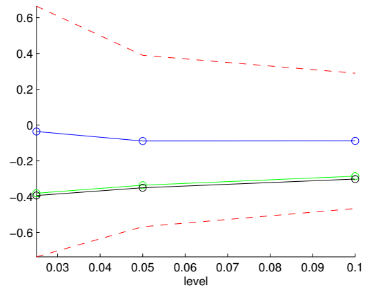
(d) lagged month average realized volatility
