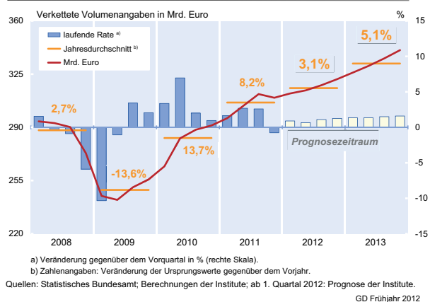
Abb. 3.3 Reale Exporte Saison- und kalenderbereinigter Verlauf
