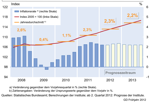
Abb. 3.8 Verbraucherpreise in Deutschland Saisonbereinigter Verlauf
