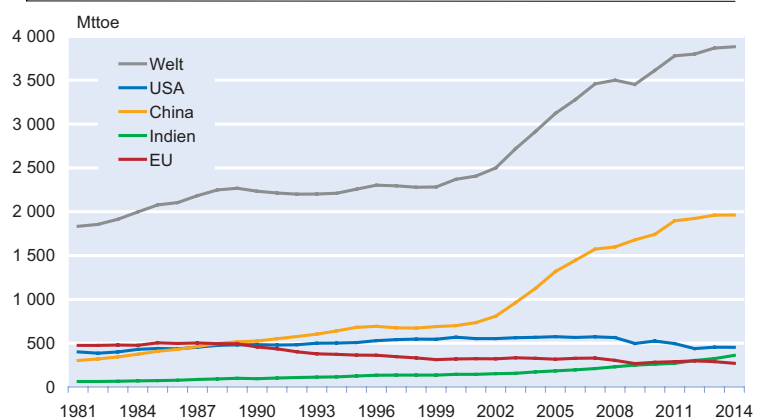
Abb. 1 Kohleverbrauch
