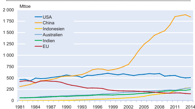
Abb. 3 Kohleproduktion
