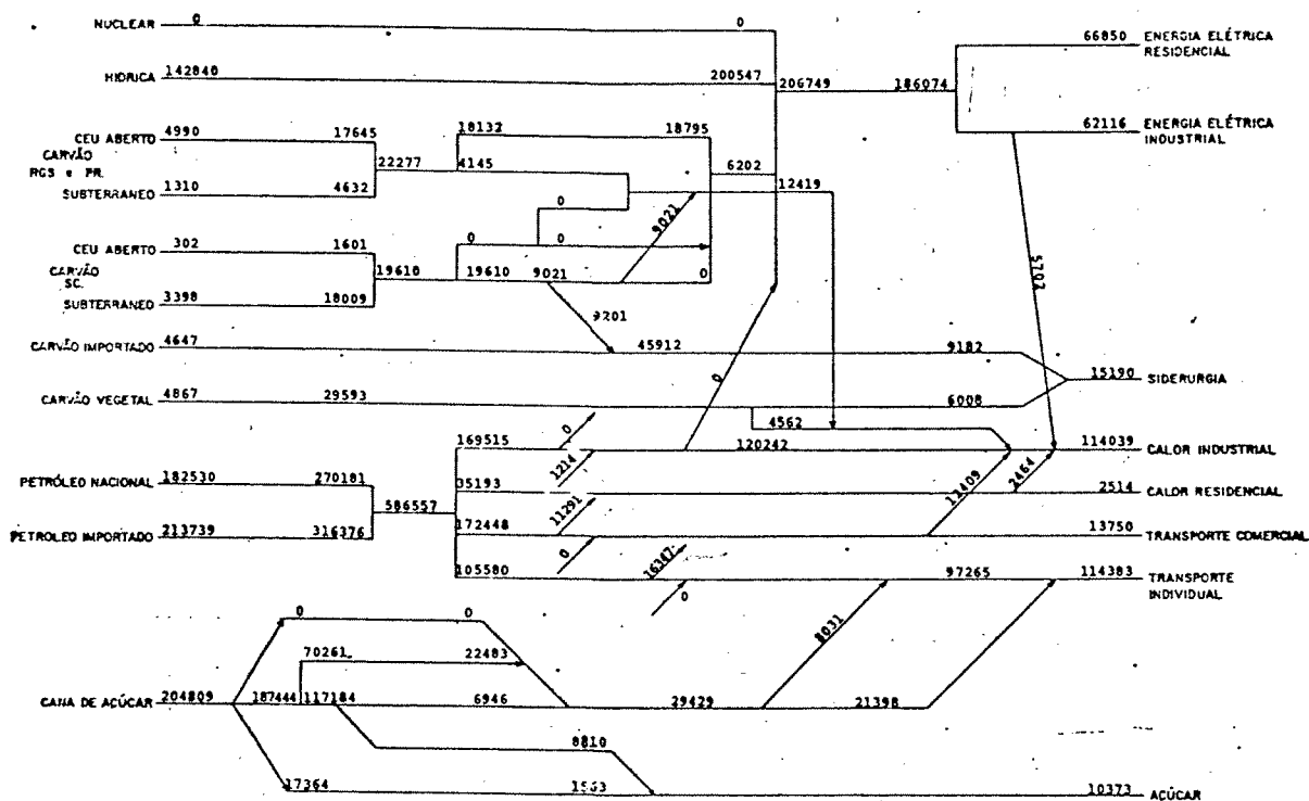
CONFIGURAÇÃO ÓTIMA DO SETOR ENERGÉTICO NACIONAL-ANO 1985 FIGURA 7
