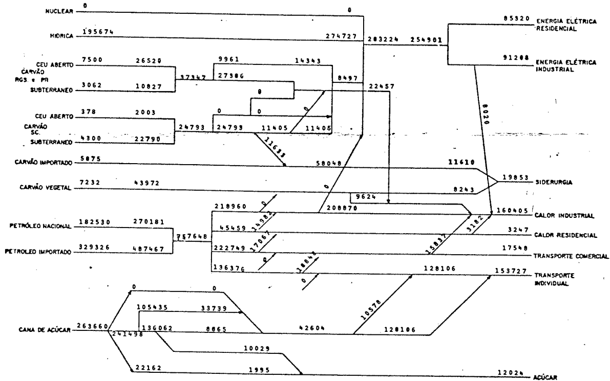
CONFIGURAÇÃO ÓTIMA DO SETOR ENERGÉTICO NACIONAL-ANO 1990 FIGURA 8
