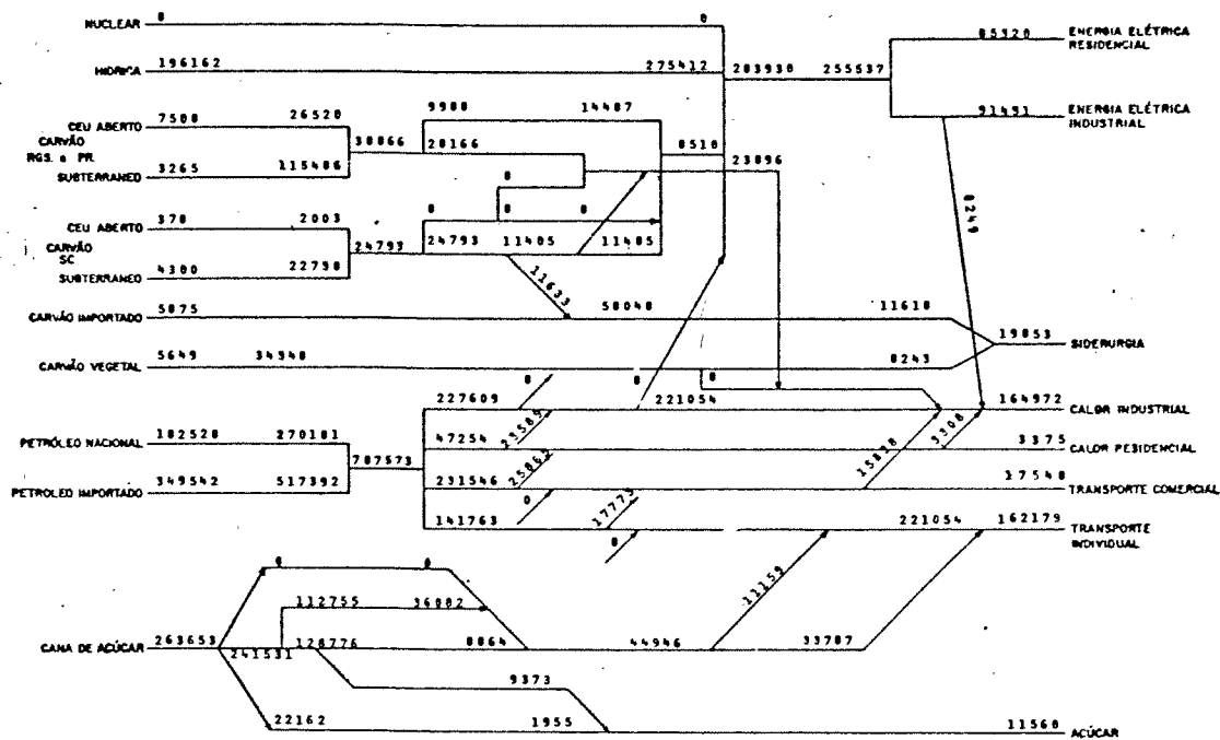
CONFIGURAÇÃO ÓTIMA DO SETOR ENERGÉTICO-ANO 1990 (CENÁRIO ALTERNATIVO B) FIGURA 10
