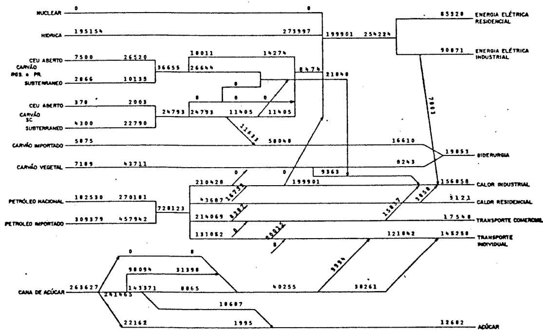
CONFIGURAÇÃO ÓTIMA DO SETOR ENERGÉTICO-ANO 1990 (CENÁRIO ALTERNATIVO A) FIGURA 9
