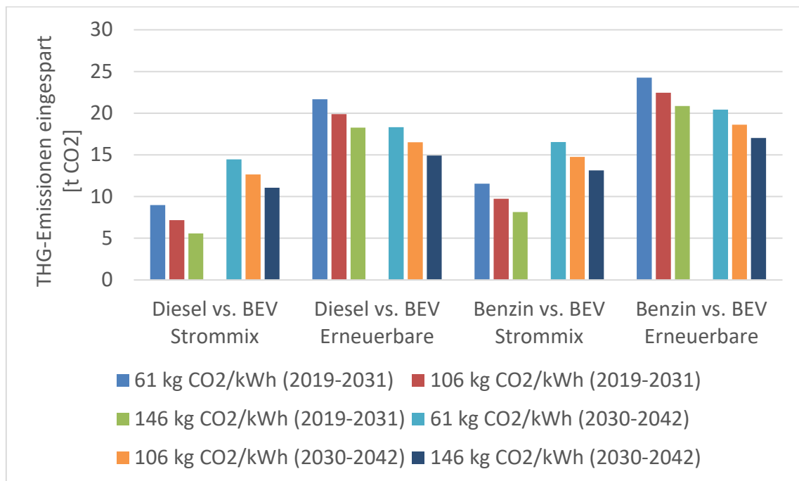
Abbildung 7: Eingesparte THG-Emissionen in Abhängigkeit der verschiedenen THG-Werte der Batterieproduktion für ein Mittelklasse-BEV mit einer Batteriekapazität von 40 kWh
