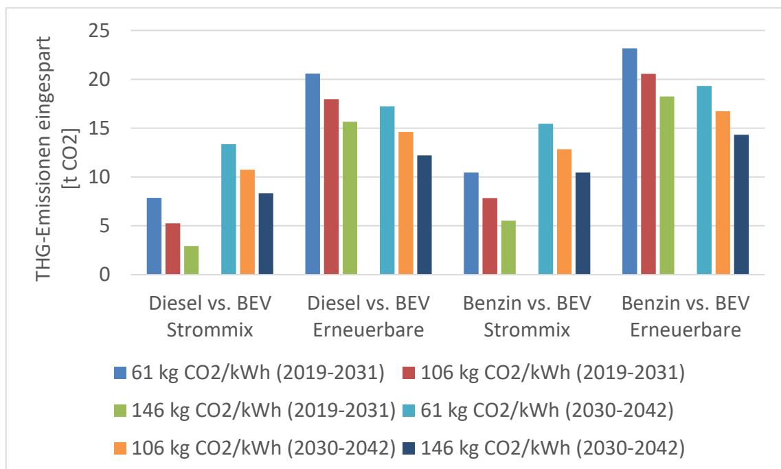
Abbildung 8: Eingesparte THG-Emissionen in Abhängigkeit der verschiedenen THG-Werte der Batterieproduktion für ein Mittelklasse-BEV mit einer Batteriekapazität von 58 kWh
