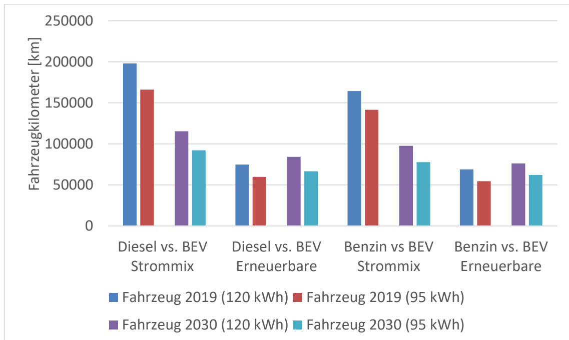
Abbildung 4: Break Even Point für ein Oberklasse-BEV mit einer Batteriekapazität von 95/120 kWh mit den THG-Emissionen bei der Batterieproduktion von 61 kg CO 2 -äq./kWh Batteriekapazität
