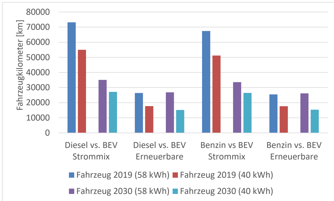
Abbildung 1: Break Even Point für ein Mittelklasse-BEV mit einer Batteriekapazität von 40 bzw. 58 kWh mit den THG-Emissionen bei der Batterieproduktion von 61 kg CO 2 -äq./kWh Batteriekapazität
