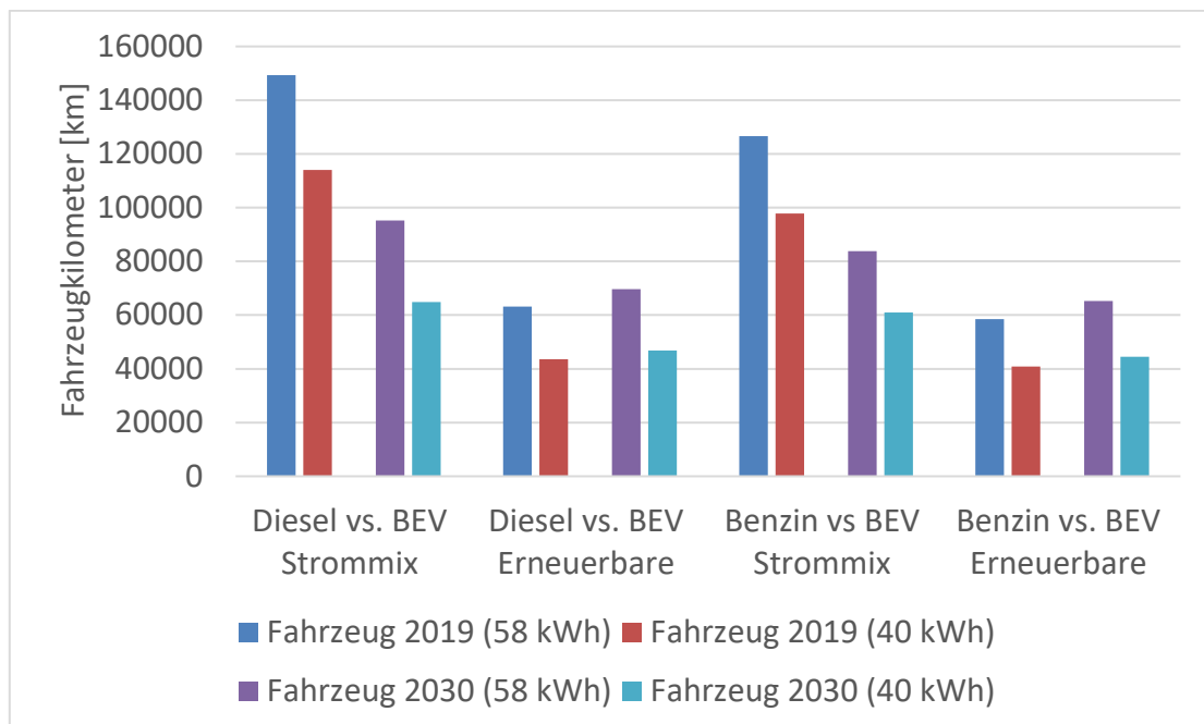
Abbildung 3: Break Even Point für ein Mittelklasse-BEV mit einer Batteriekapazität von 40 bzw. 58 kWh mit den THG-Emissionen bei der Batterieproduktion von 146 kg CO 2 -äq./kWh Batteriekapazität
