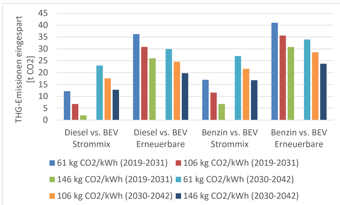
Abbildung 10: Eingesparte THG-Emissionen in Abhängigkeit der verschiedenen THG-Werte der Batterieproduktion für ein Oberklasse-BEV mit einer Batteriekapazität von 120 kWh
