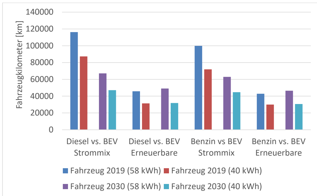
Abbildung 2: Break Even Point für ein Mittelklasse-BEV mit einer Batteriekapazität von 40 bzw. 58 kWh mit den THG-Emissionen bei der Batterieproduktion von 106 kg CO 2 -äq./kWh Batteriekapazität
