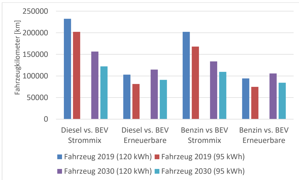
Abbildung 6: Break Even Point für ein Oberklasse-BEV mit einer Batteriekapazität von 95/120 kWh mit den THG-Emissionen bei der Batterieproduktion von 146 kg CO 2 -äq./kWh Batteriekapazität
