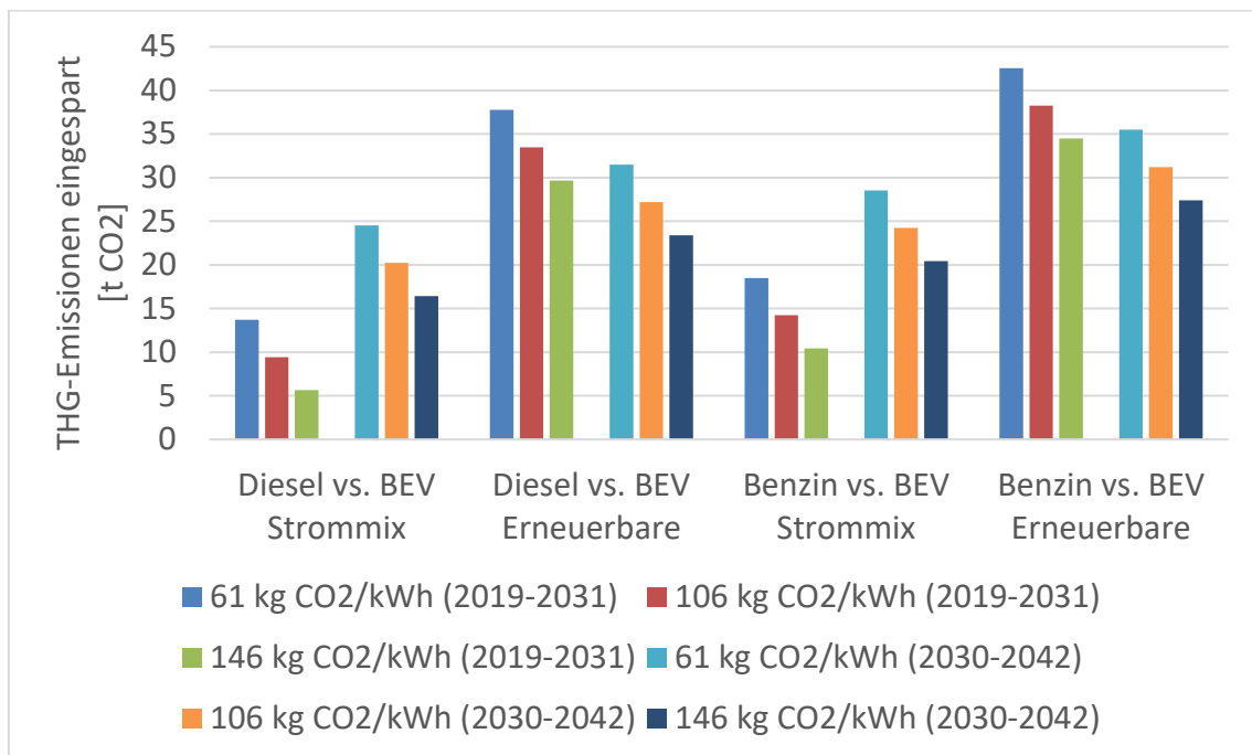
Abbildung 9: Eingesparte THG-Emissionen in Abhängigkeit der verschiedenen THG-Werte der Batterieproduktion für ein Oberklasse-BEV mit einer Batteriekapazität von 95 kWh.
