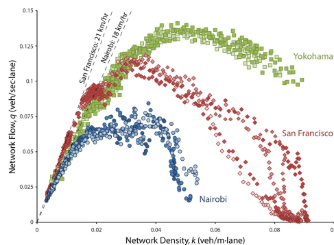
(d) Macroscopic fundamental diagram from [Daganzo et al., 2011, Fig.9].
