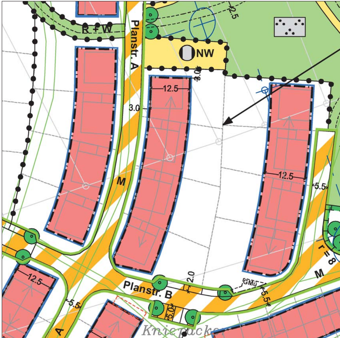
Abbildung 1: Beispiel für die Festsetzung einer Versorgungsfläche für die Nahwärmeversorgung im Bebauungsplan gemäß § 9 BauGB
