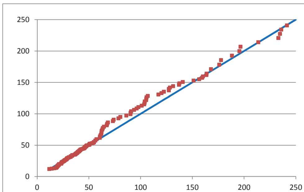
Abbildung 5: QQ-Plots der Eventschadenhöhen (3).
