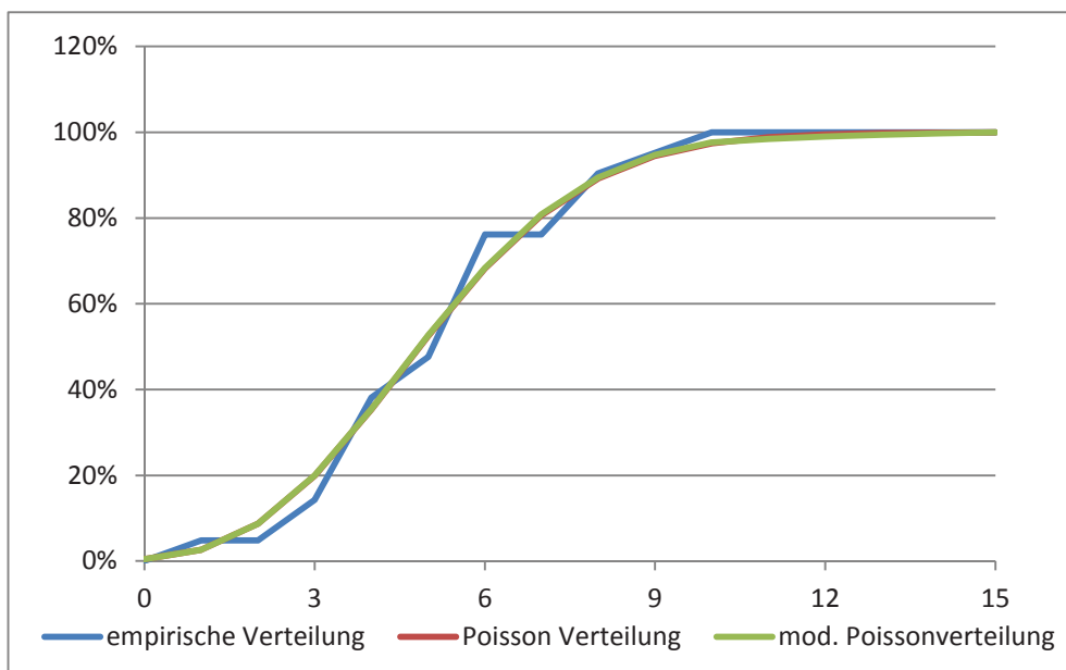
Abbildung 8: Verteilungsanpassungen für die Eventhäufigkeiten (2).
