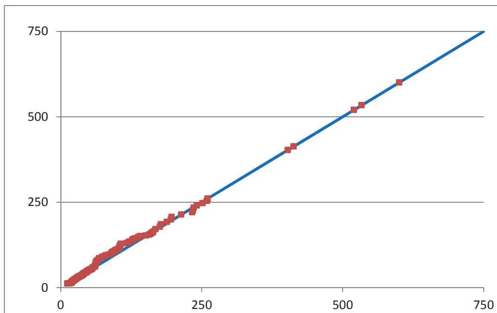
Abbildung 4: QQ-Plots der Eventschadenhöhen (2).
