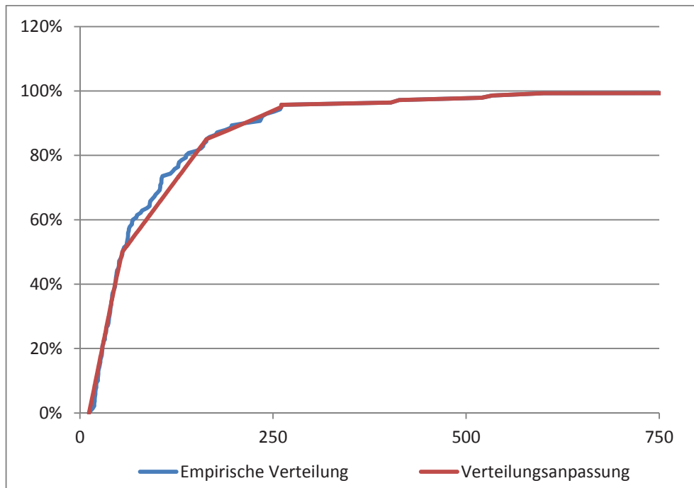
Abbildung 6: Verteilungsfunktion der Eventschadenhöhen.
