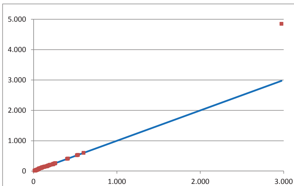
Abbildung 3: QQ-Plots der Eventschadenshöhen (1).
