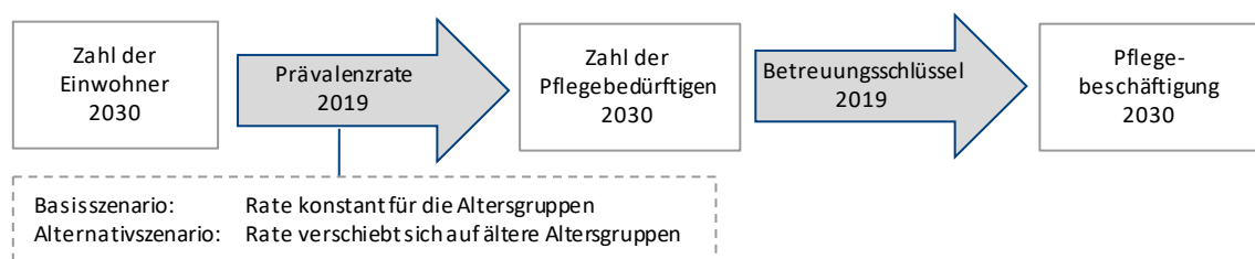
Abbildung 2: Schematischer Aufbau der Modellrechnungen zum nachfragebedingten Erweiterungsbedarf
