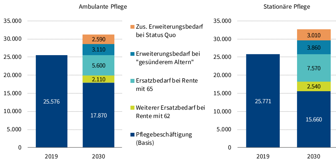
Abbildung 9: Beschäftigungsbedarf in Schleswig-Holstein bis 2030 in Vollzeitäquivalenten
