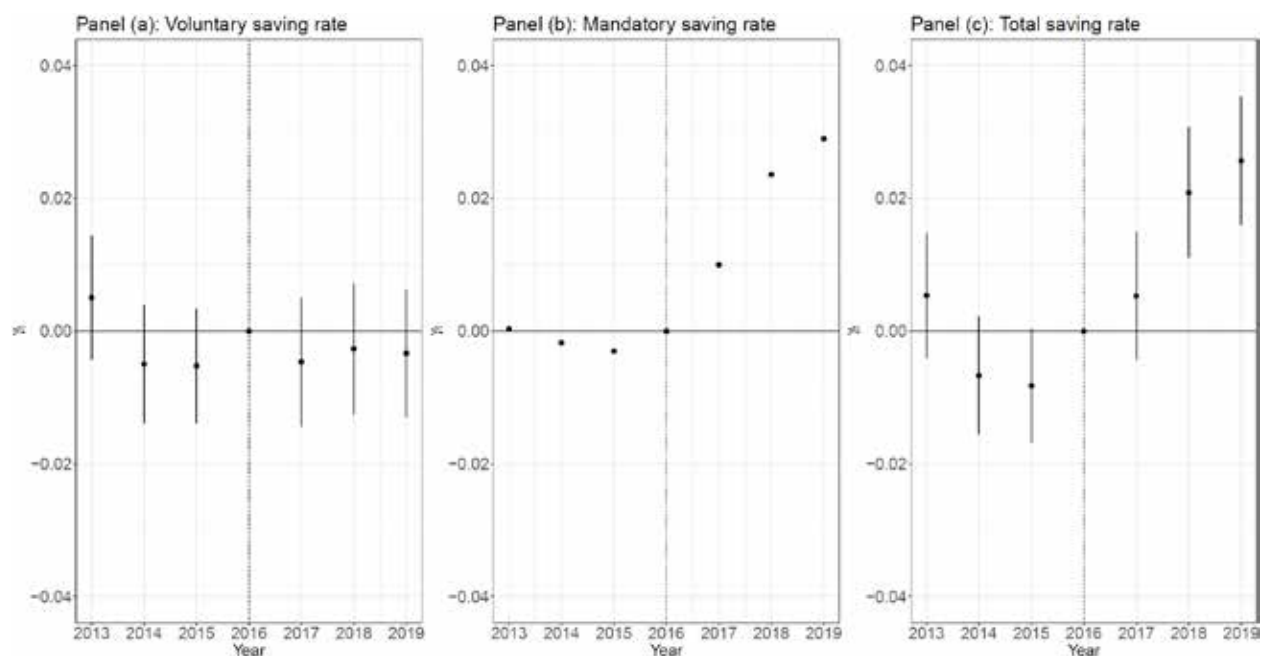
Figure A5-2: Estimates of parameter \gamma_t
