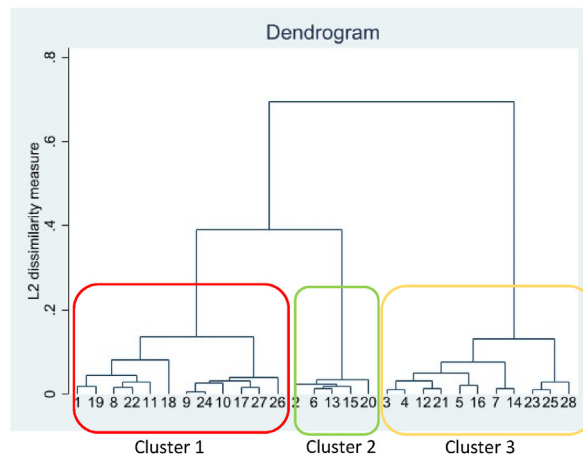
Fig. 3. Dendrogram.
