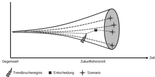
Abbildung 7: Szenario-Trichter 43
