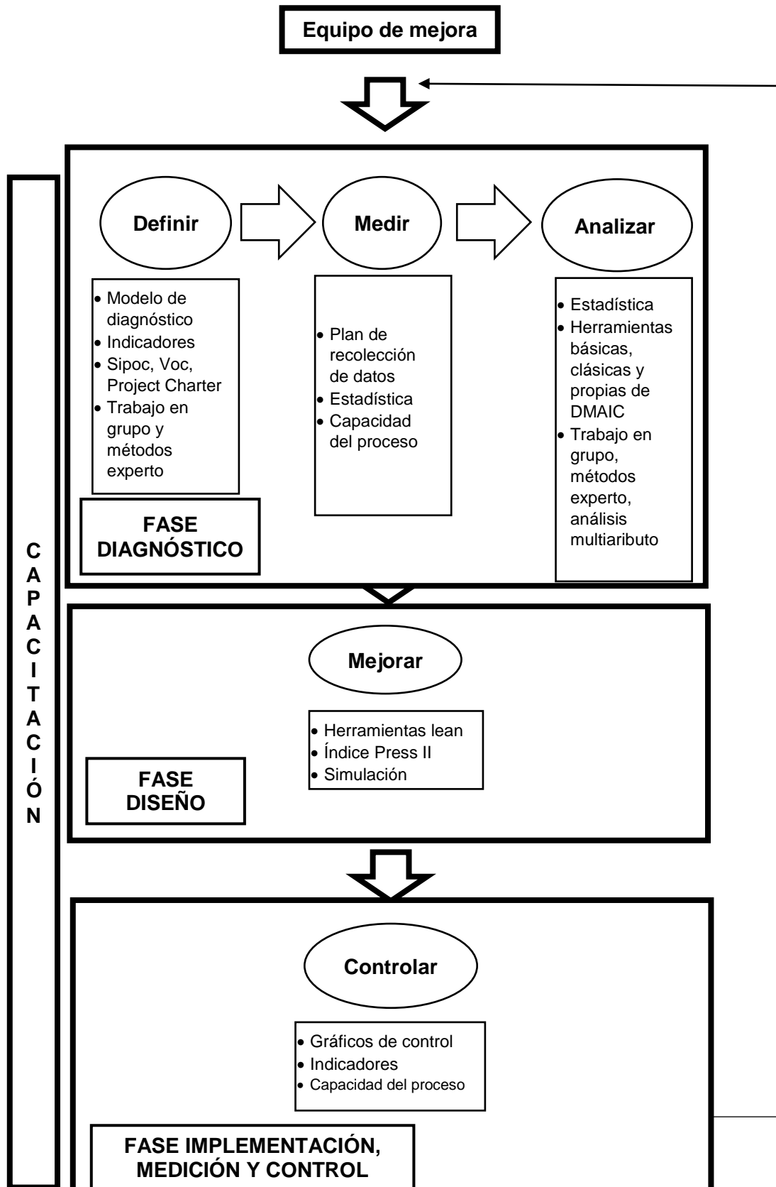
Figura 1: Modelo basado en las metodologías Lean, Seis Sigma y herramientas cuantitativas.
