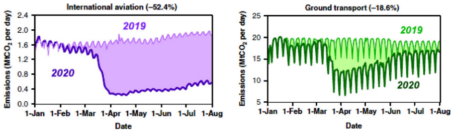
Abb. 1 Weltweiter CO 2 -Ausstoß im internationalen Flugverkehr sowie im Straßenverkehr im ersten Halbjahr 2020 verglichen mit dem Vorjahreszeitraum. Quelle: Liu et al. (2020)
