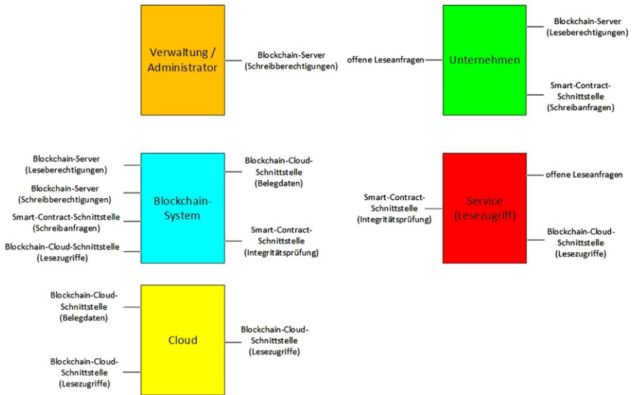
Abb. 1 Module mit eingehenden linken und ausgehenden rechten Schnittstellen des Lösungskonzepts
