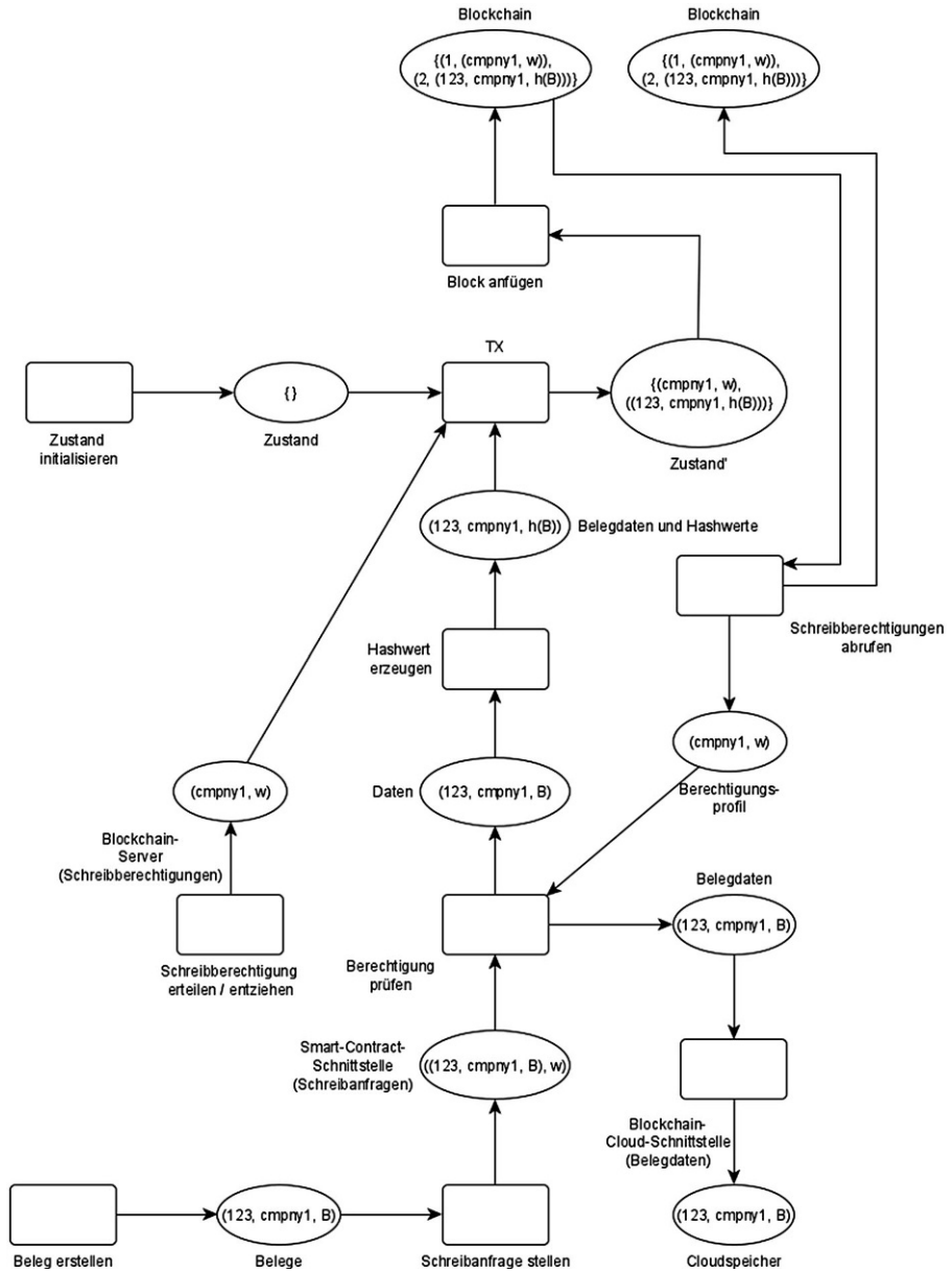
Abb. 3 Verteilter Ablauf der Erfassung eines Belegs
