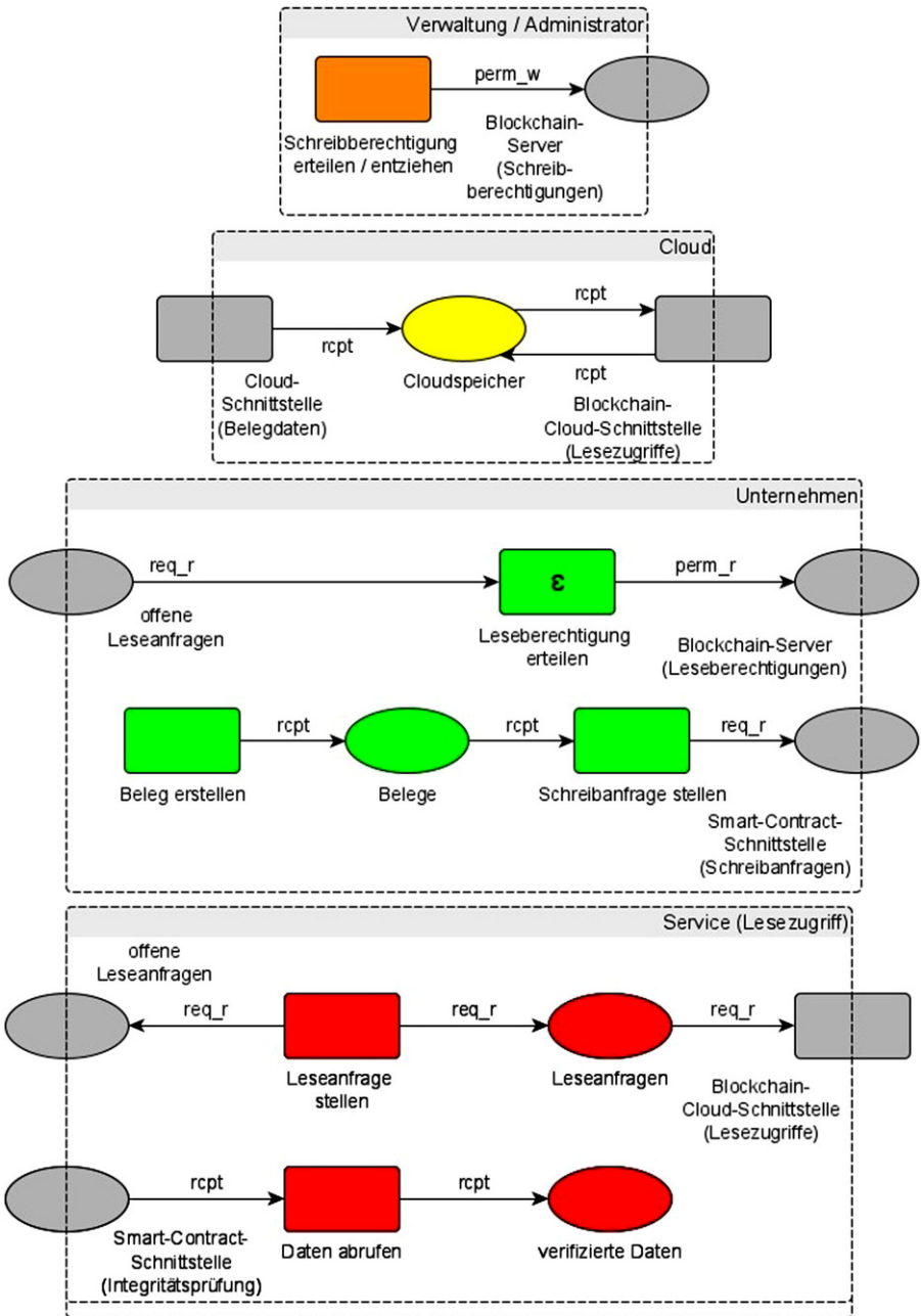
Abb. 5 Modularisierte Darstellung des Systems zur Erfassung von Belegen und Standard Audit Files
