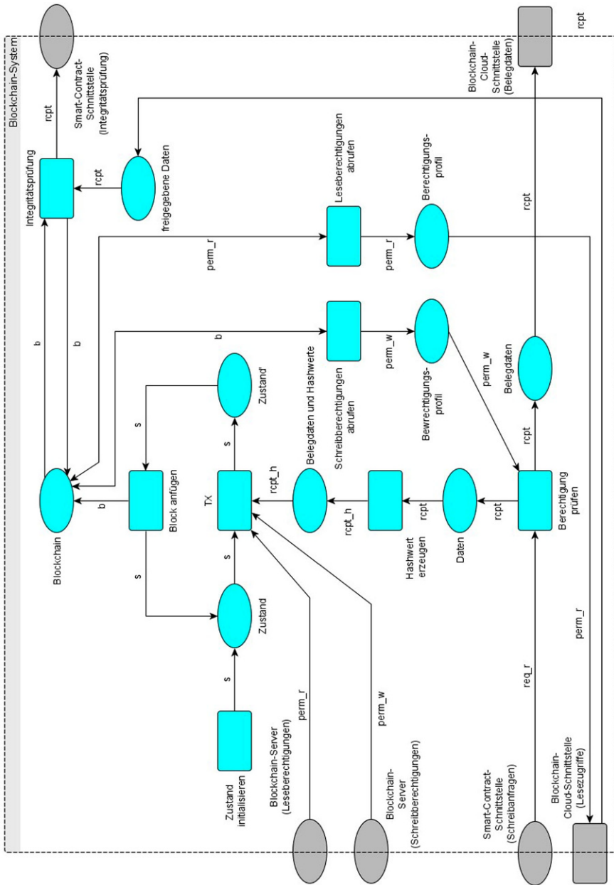
Abb. 2 Modularstellung der Blockchain-Komponente
