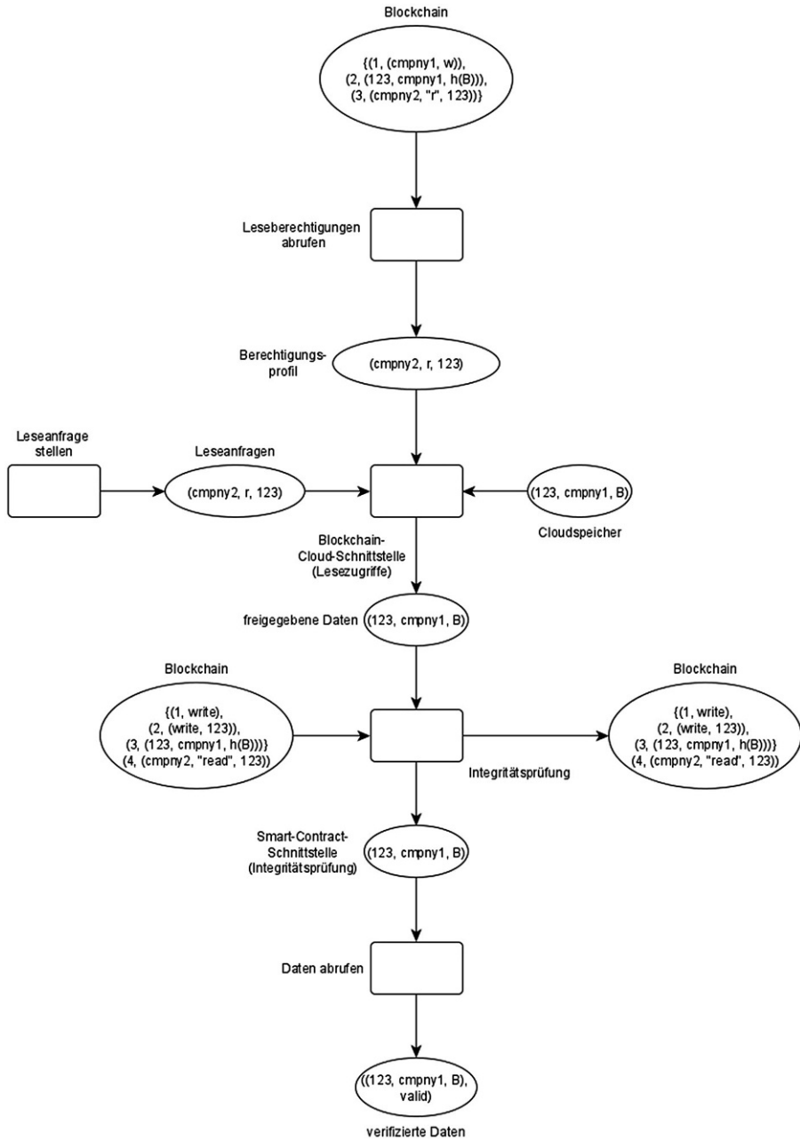
Abb. 4 Verteilter Ablauf des Lesezugriffs auf einen Beleg sowie dessen Verifikation
