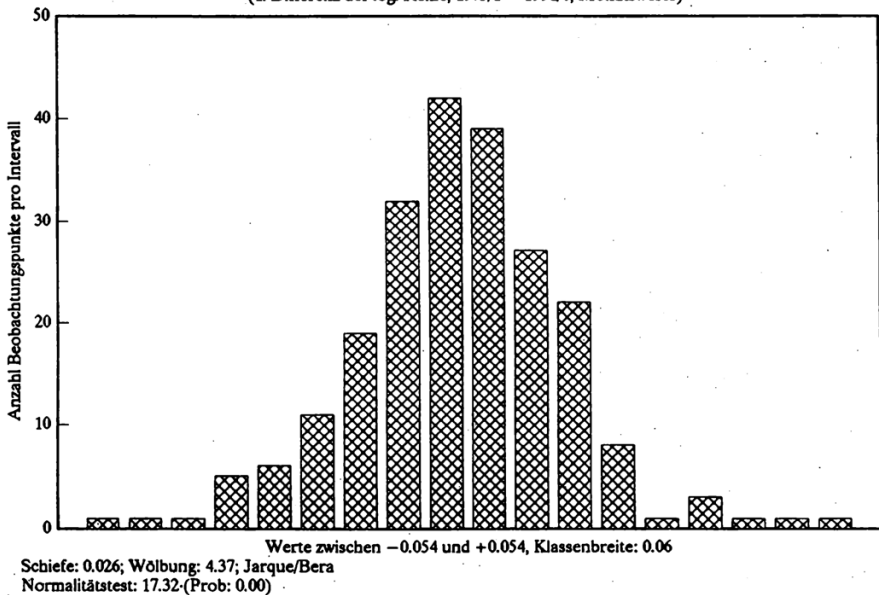
Abb. 2 Histogramm SFr/DM–Wechselkurs
