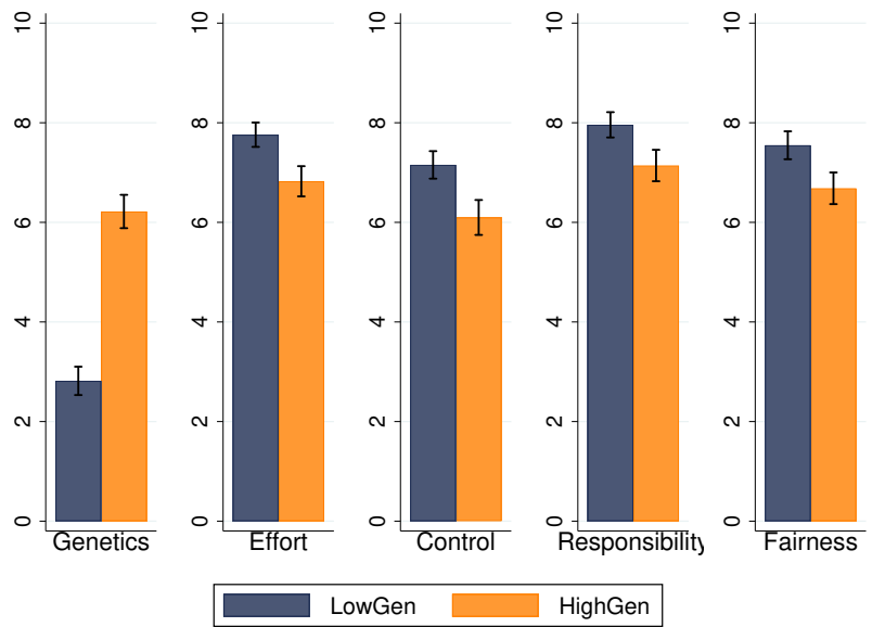
Figure 2: Posterior Beliefs
