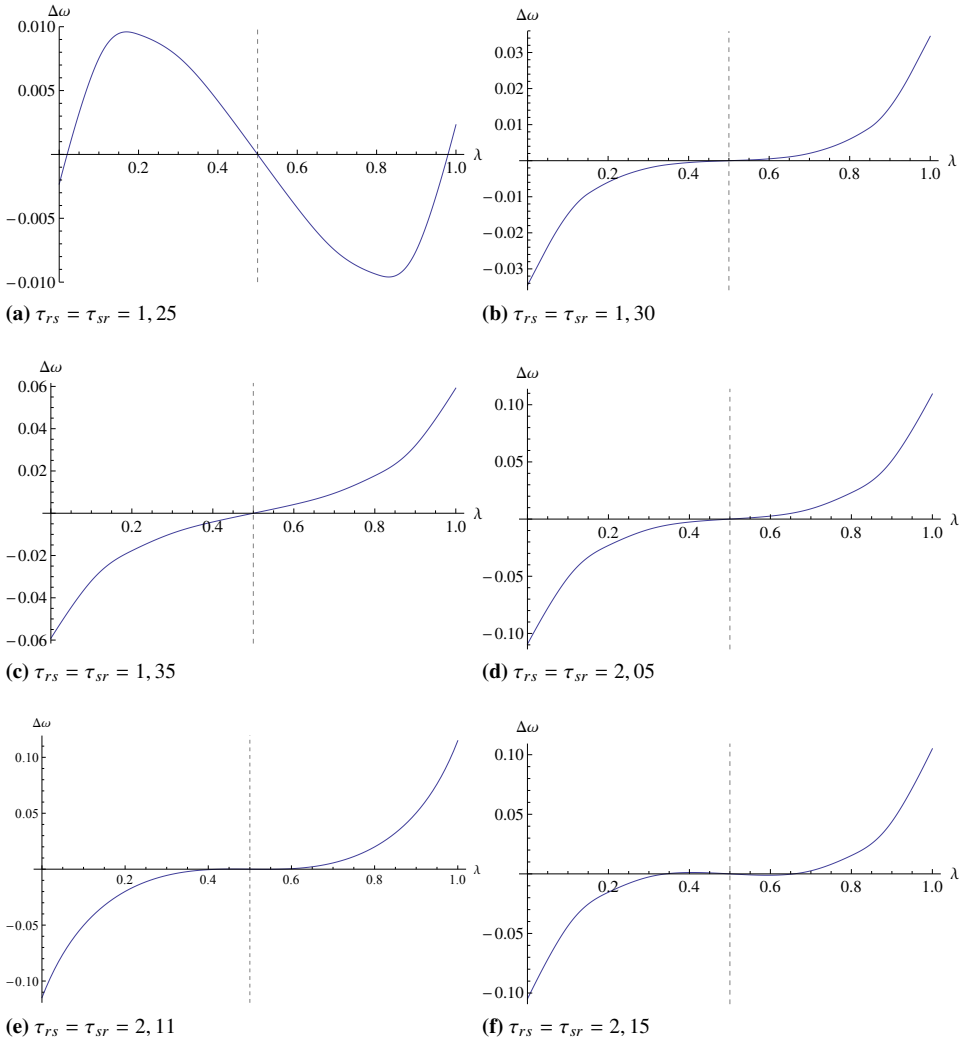
Abbildung 4.1.4: Visuelle Bestimmung der Breakpoints am Beispiel gleich großer Regionen
