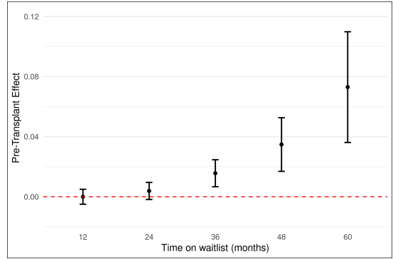
(d) Post-2015
