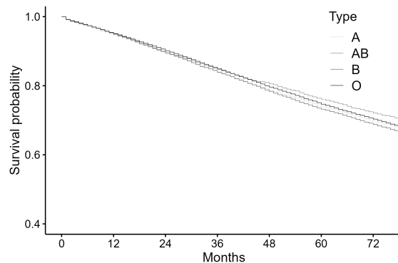
(d) Survival
