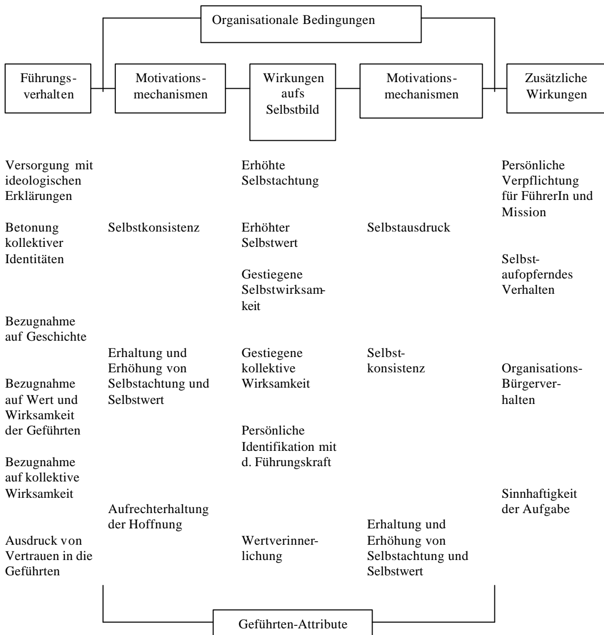
Abbildung 2: Skizze der Theorie nach Shamir, House&Arthur; 1996, 218 (zit. n. Neuberger; 2002, S. 167)
