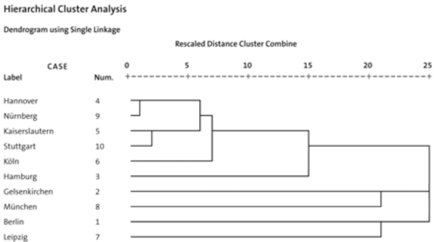
Abb. 8: Clusteranalyse (Ward-Verfahren)
