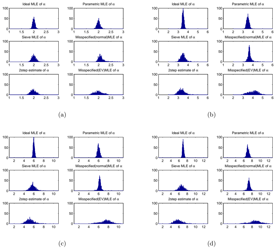
Figure 6: Gumbel copula : Histograms of \alpha estimates (a) true \alpha=2 , (b) true \alpha=3.5 , (c) true \alpha=6 , (d) true \alpha=7
