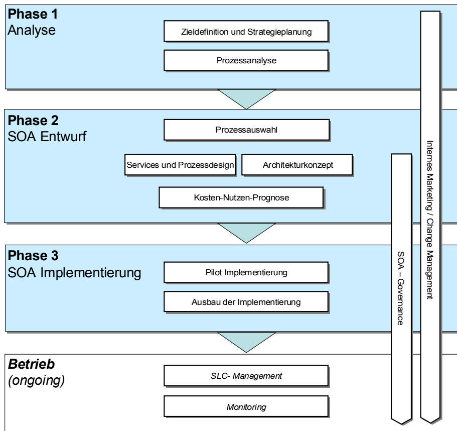
Abbildung 2: SOA Vorgehensmodell
