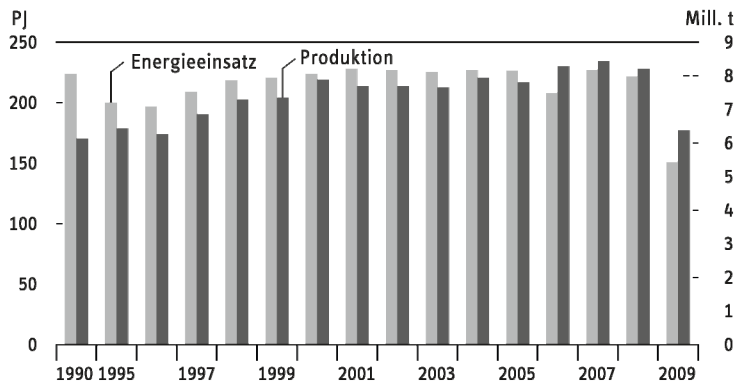
Schaubild 13.1 Produktion und Energieverbrauch der NE-Metallindustrie 1995 bis 2009
