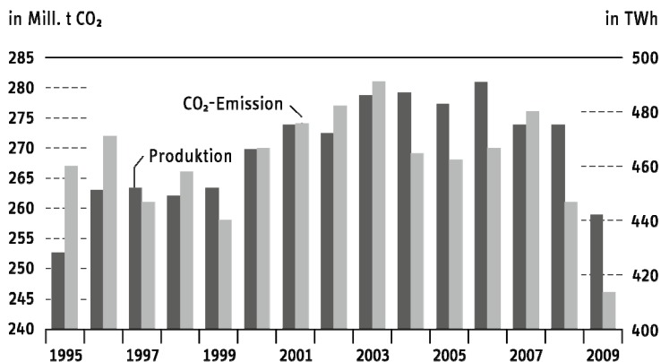
Schaubild 19.1 CO 2 -Emissionen und Nettostromerzeugung der allgemeinen Elektrizitätswirtschaft 1995 bis 2009; ohne umgruppierte Industriekraftwerke und Deutsche Bahn
