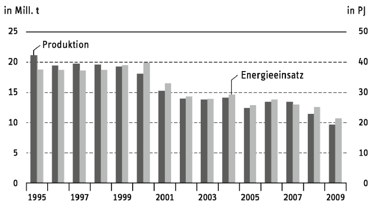
Schaubild 9.1 Produktion und Energieverbrauch in der Ziegelindustrie 1995 bis 2009
