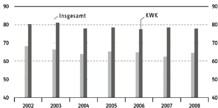
Nutzungsgrade der industriell betriebenen Strom- und Wärmeerzeugungsanlagen 2002 bis 2008, in %
