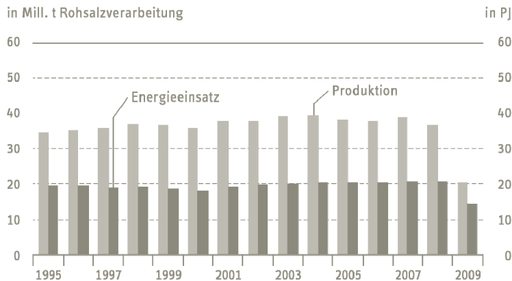
Schaubild 1.1 Produktion und Energieeinsatz der Kaliindustrie 1995 bis 2009
