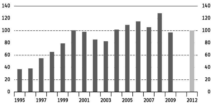
Schaubild 14.3 Zielerreichungsgrad der Elektroindustrie für das Minderungsziel 2012 1995 bis 2009; in %
