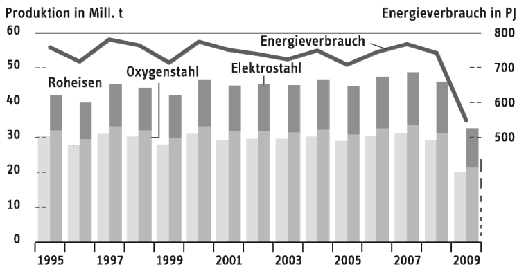
Schaubild 12.2 Produktion und Nettoenergieverbrauch in der Stahlindustrie 1995 bis 2009
