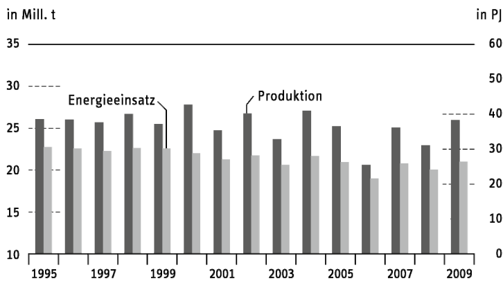
Schaubild 2.2 Energieverbrauch und Rübenverarbeitung in der Zuckerindustrie 1990 bis 2009
