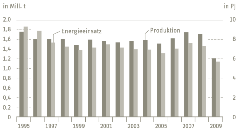
Schaubild 7.2 Produktion und Energieverbrauch in der Feuerfest-Industrie 1995 bis 2009
