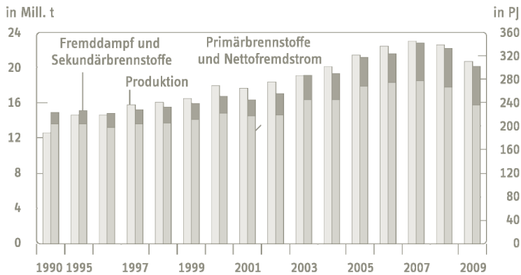
Schaubild 4.2 Produktion und Energieeinsatz in der Papierindustrie 1990 bis 2009
