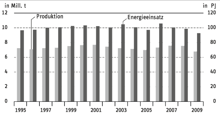
Schaubild 6.2 Produktion und Energieverbrauch in der Glasindustrie 1995 bis 2009
