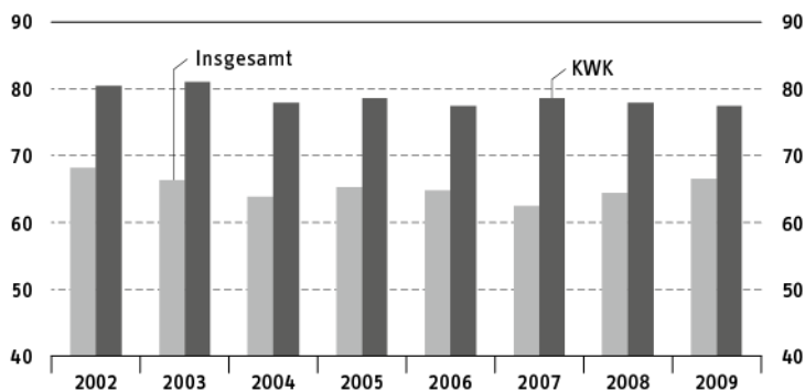
Schaubild 18.1 Nutzungsgrade der industriell betriebenen Strom- und Wärmeerzeugungsanlagen 2002 bis 2009, in %
